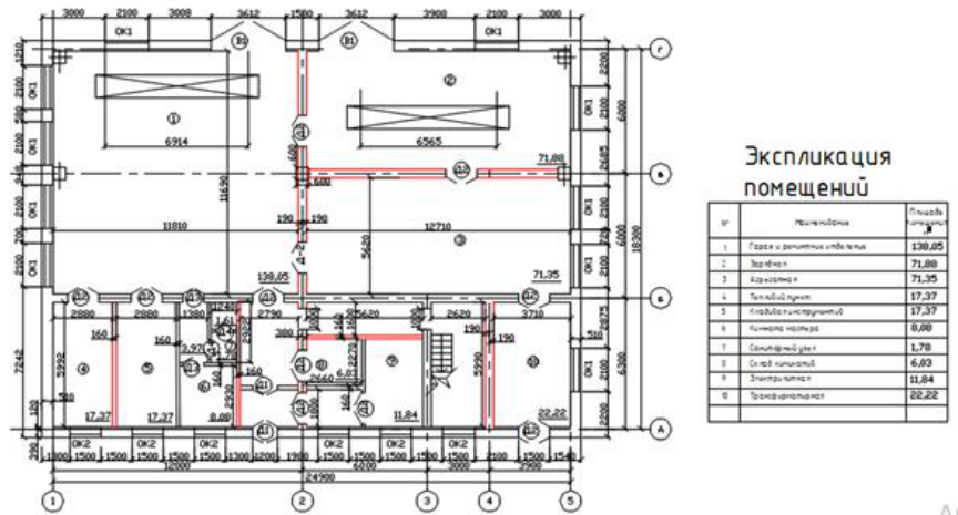
План 1-го этажа М 1:100
